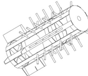
Gambar 6. Rancangan Roda
