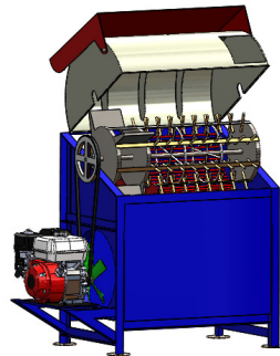
Gambar 7. Rancangan Mesin Perontok Sistem Lorong Hembus
