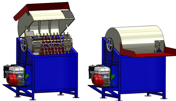
Gambar 4. Rancangan Mesin Perontok Padi Sistem Lorong Hembus
