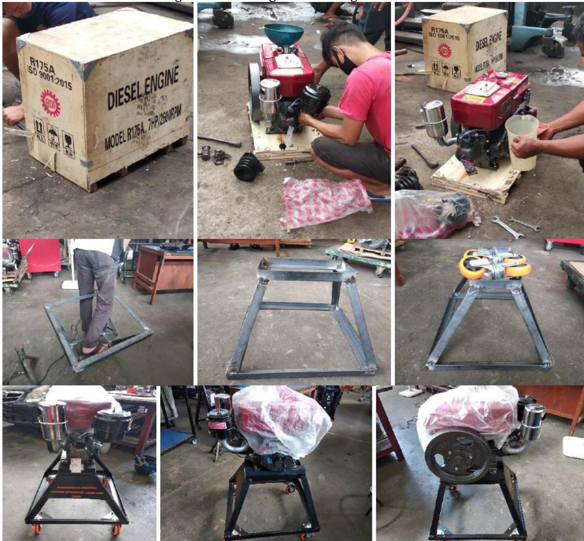
Gambar 1. Proses pembuatan stand , perakitan dan pemasangan mesin.
